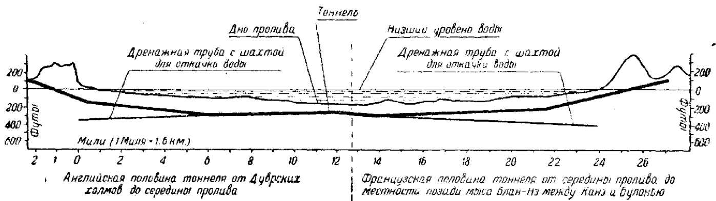
Схема проекта тоннеля под Ламашем.
